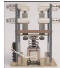
E25-2PDT-25 Low Profile
